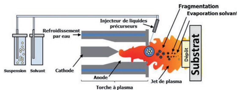
Schéma de principe du procédé SPS
