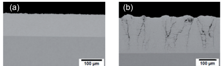
Exemples de microstructures de revêtements obtenues par SPS avec (a) ou sans (b) filtrage sélectif des gouttelettes.
