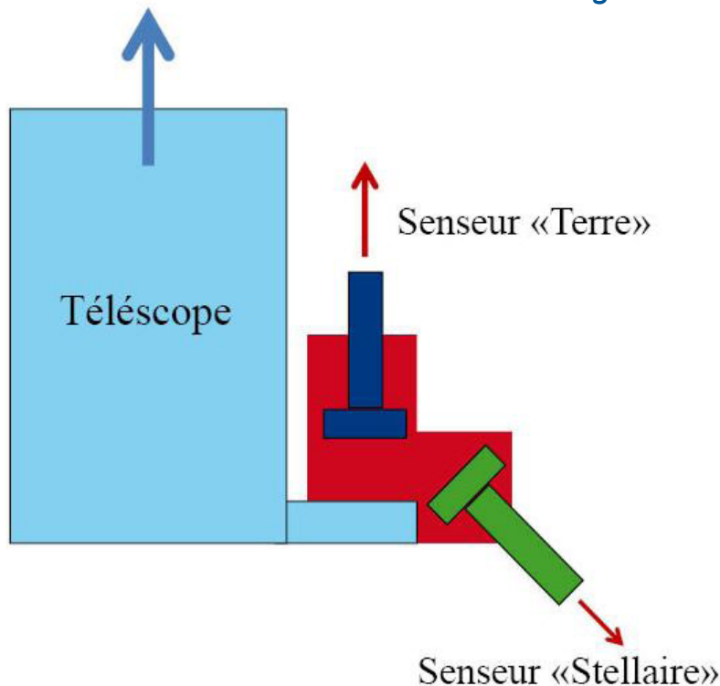
Principe d'acquisition
