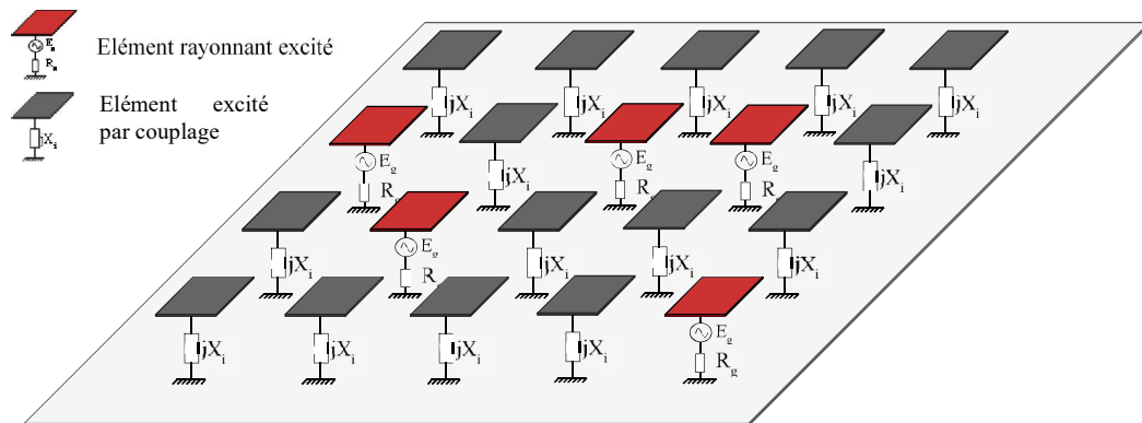
Figure 1 : Schéma de principe de l'antenne hybride – Éléments excités (en rouge) et éléments non excités chargés par des impédances complexes (en gris)
