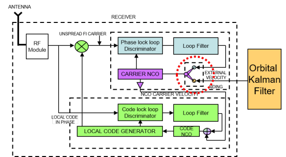
Algorithme spécifique de poursuite des ondes porteuses
